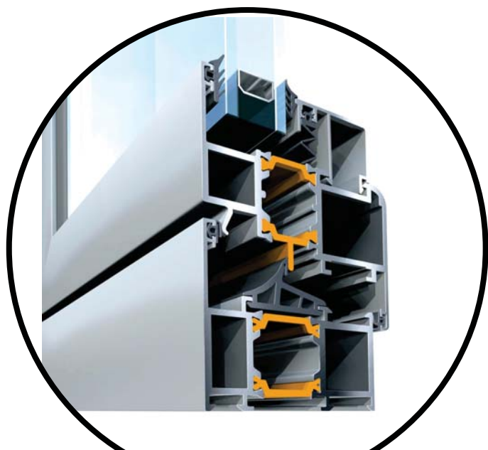
SMARTIA M11000 -alumil-
