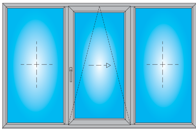
deschidere oscilo-culisantă
