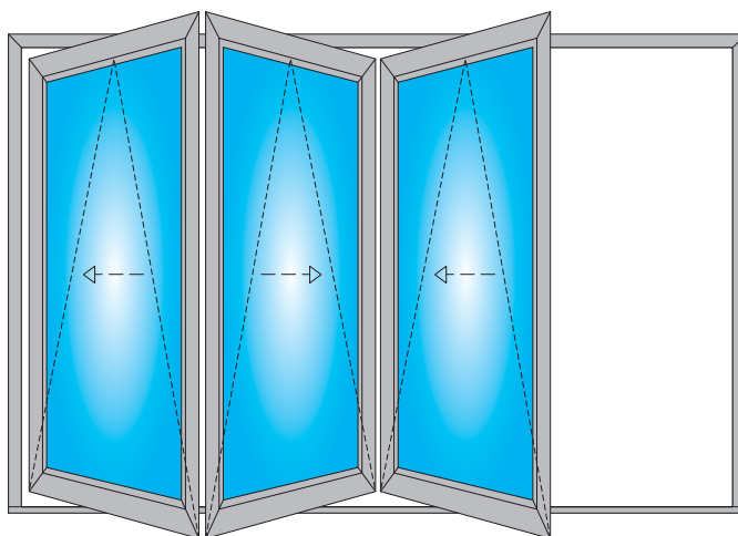
deschidere armonică
