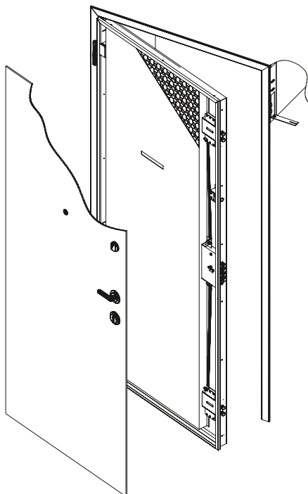
Desen tehnic pentru usa intr-un canal
