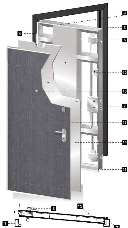
Desen tehnic pentru usa intr-un canal
